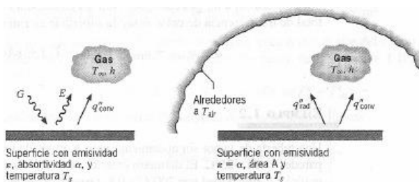
Imagen 2. Radiación en la superficie. Radiación entre una superficie y sus alrededores.
