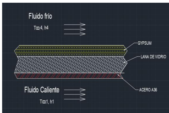
Imagen 5. Esquema del circuito de Resistencia Térmica para inferior
