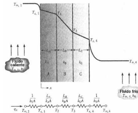
Imagen 9. Circuito térmico equivalente para una pared compuesta en serie. Fuente:( Frank Incropera, 2000)
