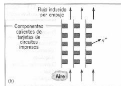
Imagen 4. Convección Natural. Fuente:( Frank Incropera, 2000)
